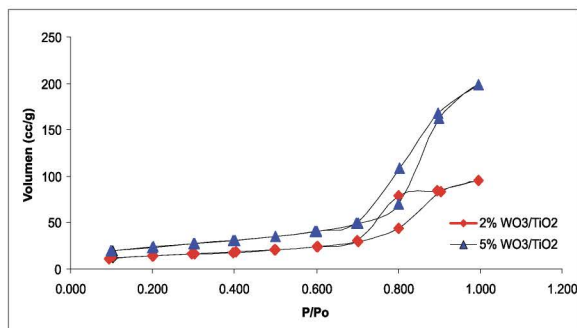
Figura 6. Isotermas de adsorción-desorción de N 2 del WO 3 /TiO 2 sintetizado por sol-gel.
