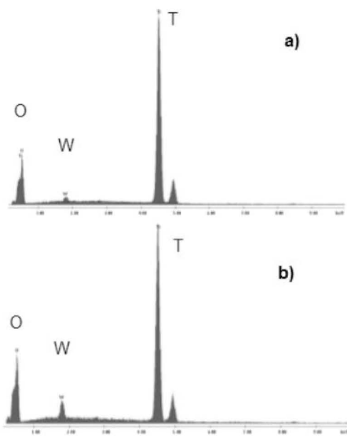
Figura 5. Análisis EDAX del óxido mixto a) WO 3 /TiO 2 - 2% y b) WO 3 /TiO 2 al 5% sintetizado por sol-gel.
