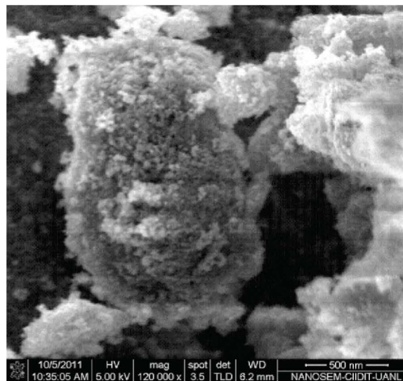
Figura 3. Imagen SEM del WO 3 /TiO 2 -2% sintetizado por sol-gel (Medida de referencia 500nm).
