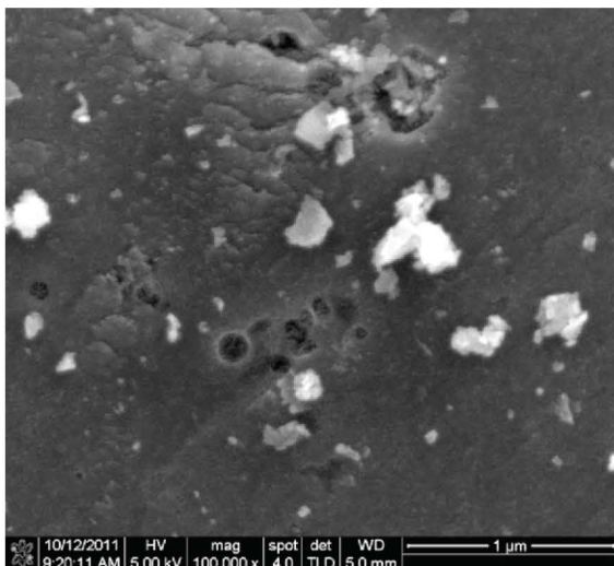
Figura 4. Imagen SEM del WO 3 /TiO 2 al 5% sintetizado por sol-gel. (Medida de referencia 1 μm).
