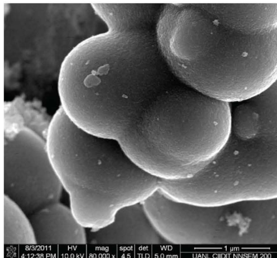
Figura 2. Imagen SEM de TiO 2 sintetizado por sol-gel (Medida de referencia 1μm).
