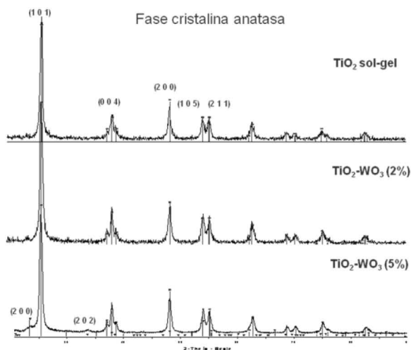
Figura 1. Patrones de DRX del TiO 2 y TiO 2 -WO 3 (2 y 5%) sintetizados por sol-gel.
